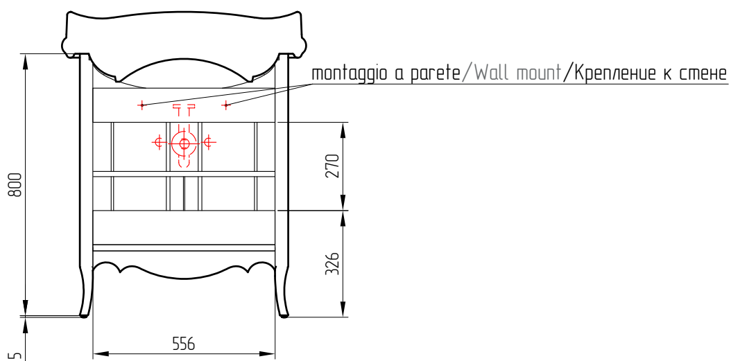
Vista posteriore/Rear view/Вид сзади
